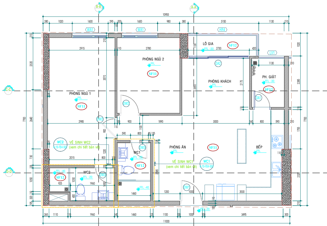
MẶT BẰNG KÍCH THƯỚC TL:1/50
